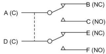
Double Pole (DPDT)
